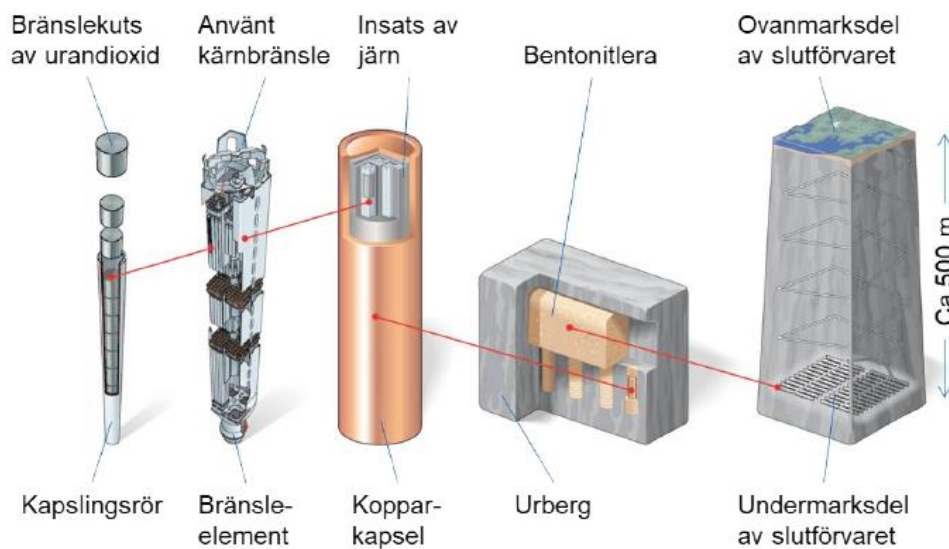
Figur 1-2. KBS-3-metoden.
